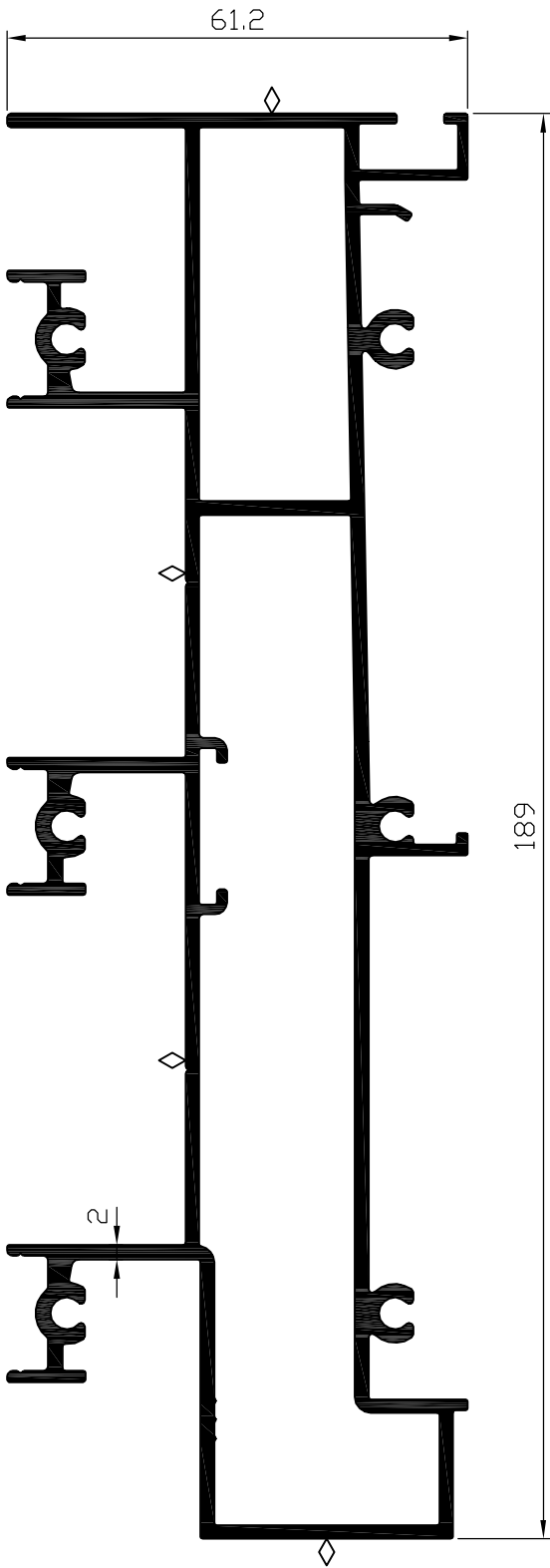
מסילה תחתונה 61 מ"מ 3 נתיבים 06262 פרופיל משקל : 3647 מ"ג היקף כללי : 1465 מ"מ היקף חיצוני : 977 מ"מ
