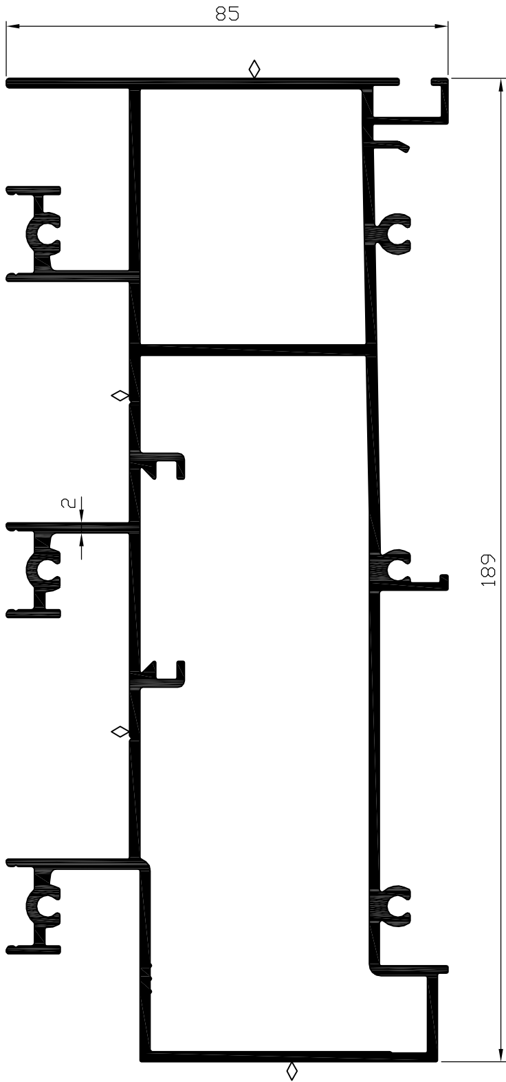
מסילה תחתונה 85 מ"מ 3 נתיבים 07461 פרופיל משקל : 4367 מ"ג היקף כללי : 1637 מ"מ היקף חיצוני : 1025 מ"מ
